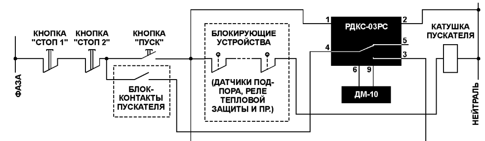
Рис. 5. Пример включения РДКС-03 в схему блокировки автономного конвейера.
