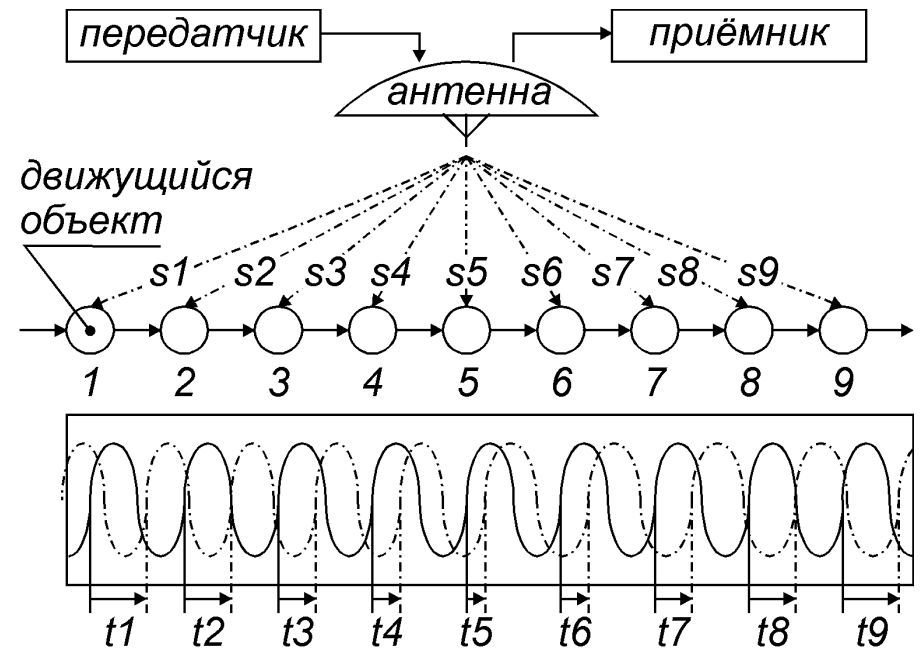
Рис. 3. Эффект Доплера.
